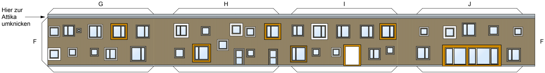
Fassaden Haus 2
